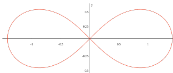
Analema 1 del Sol y Lemniscata 2 en geometría analítica, respectivamente
