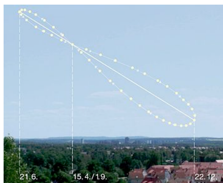
Analema 1 del Sol y Lemniscata 2 en geometría analítica, respectivamente
